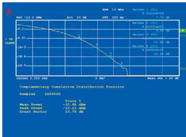
WCDMA信号的CCDF功能
